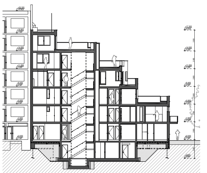
Řez A-A
