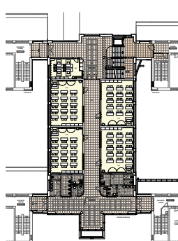
PŮDORYS 2.NP 1:250
