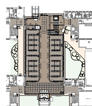
PŮDORYS 1.NP 1:250
